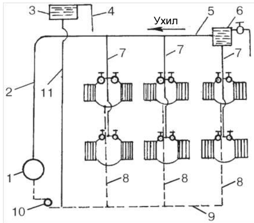
Малюнок 16. Системи водяного опалення з примусовою циркуляцією (верхня розводка) 1 — котел; 2 — головний стояк; 3 — розширювальний бак; 4 — сигнальна лінія; 5 — лінія, що подає; 6 — повітрозбирач; 7 — стояки, що подають; 8 — зворотні стояки; 9 — зворотна лінія; 10 — насос; 11 — розширювальна труба
