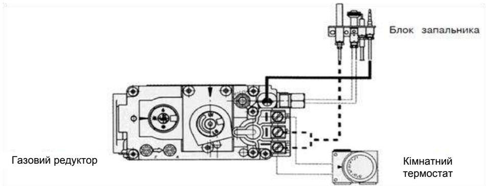
Малюнок 9. Схема зовнішніх з'єднань газового редуктора
